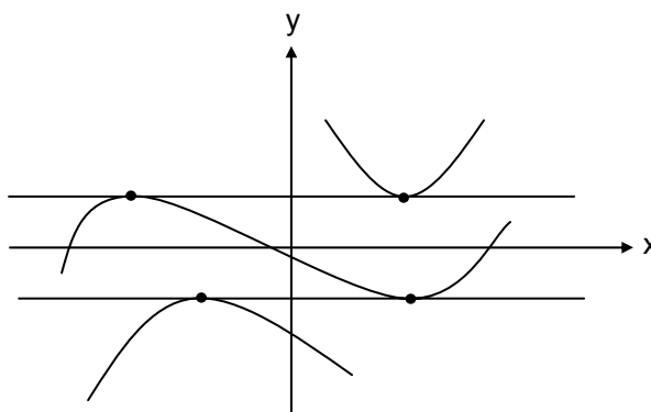
Recta con pendiente 'cero'
