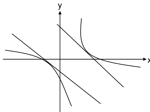
Recta con pendiente negativa
